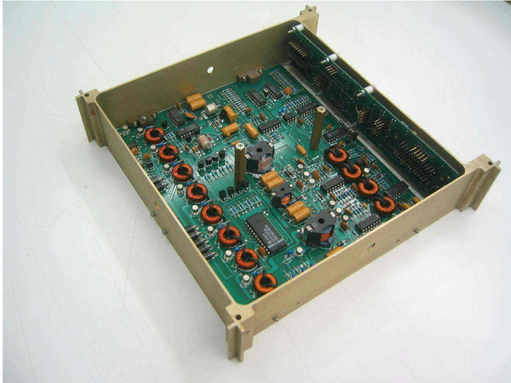
Módulo de alimentación de los satélites, diseñado y construido en Chile
